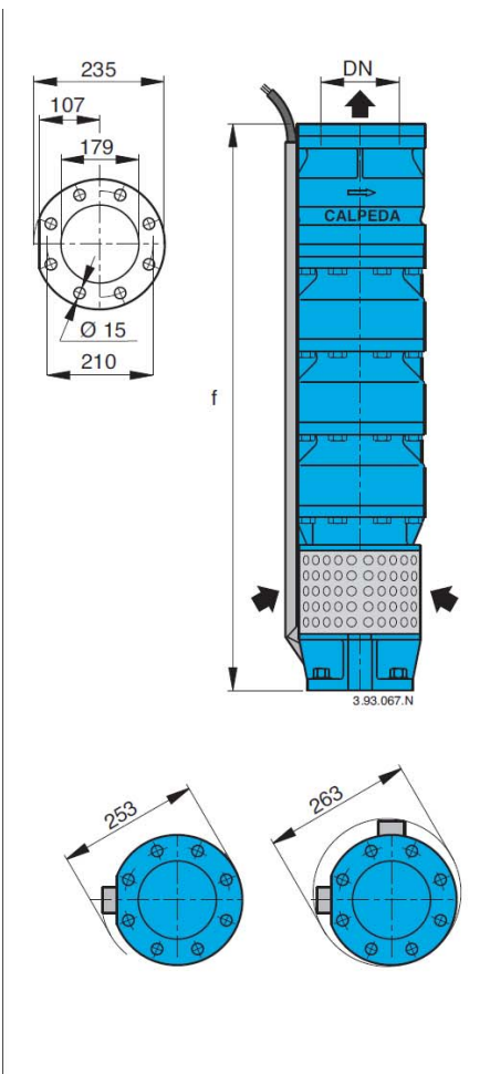
Hegeszthető ellenkarima
